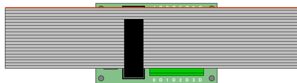
Figuur 11: Aansluiten SWdec op een 20-polige SHdec kabel
