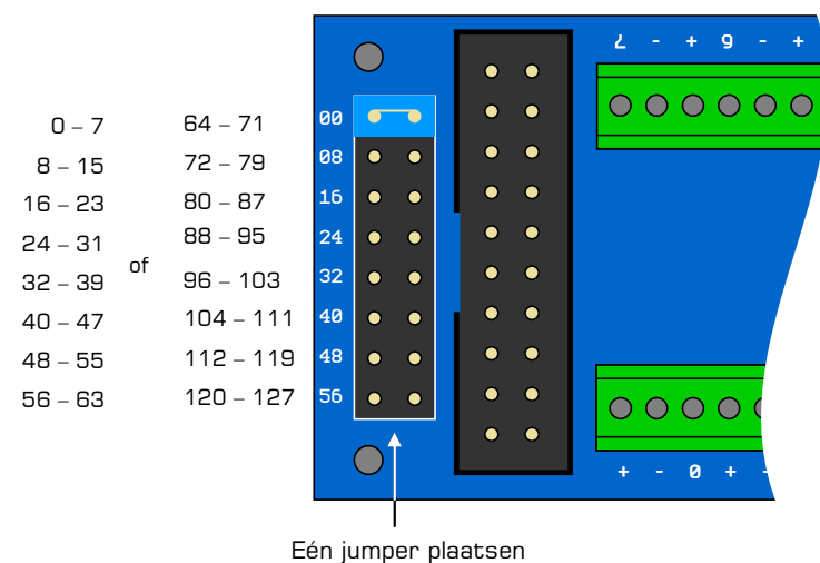
Figuur 7: SHdec adres selectie
