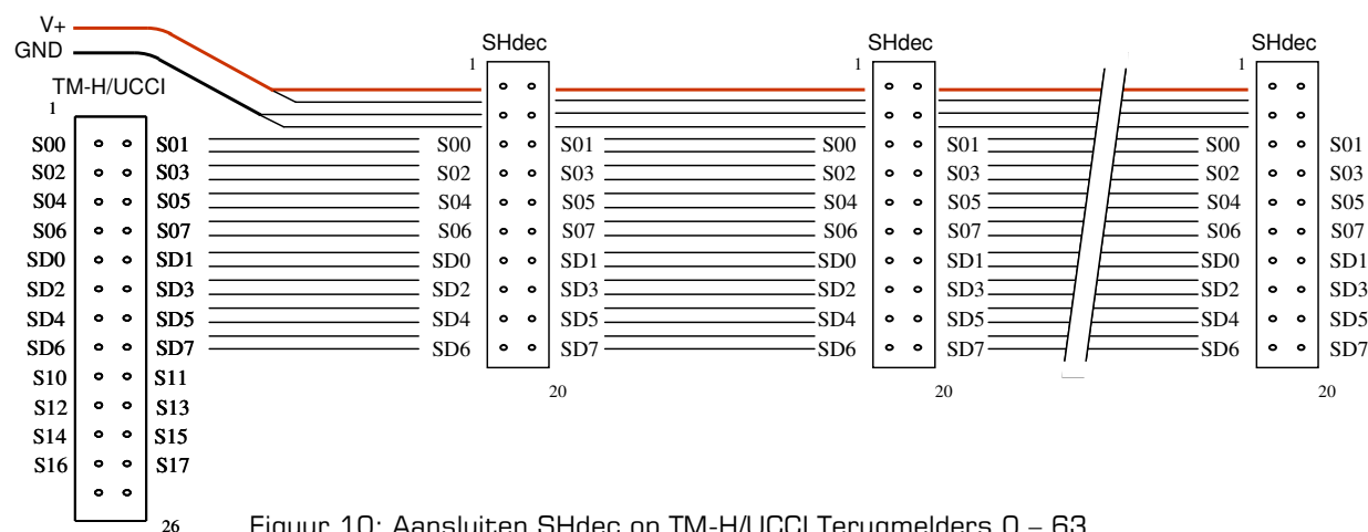
Figuur 10: Aansluiten SHdec op TM-H/UCCI Terugmelders 0 – 63
