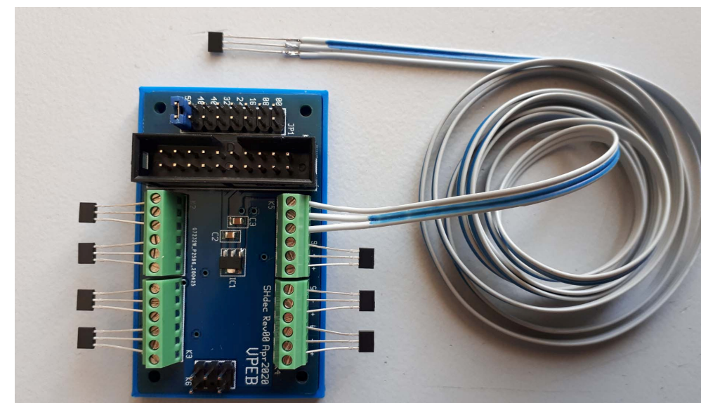
Figuur 6: Voorbeeld gebruik gekleurde bandkabel om sensor-draden te verlengen
