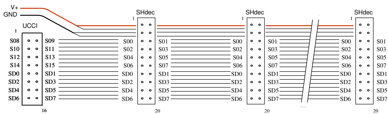
Figuur 11: Aansluiten SHdec op UCCI Terugmelders 64 - 127
